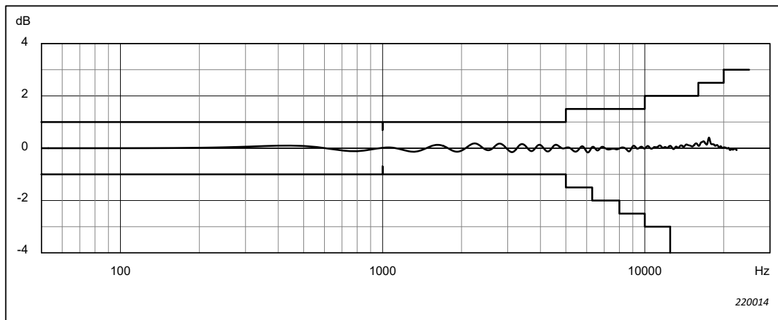
Abb. 4.5 0°-Freifeld-Frequenzgang für Mikrofon Typ 4966, Mikrofonvorverstärker ZC-0043 und den Schallpegelmesser, wenn der Mikrofonvorverstärker direkt am Schallpegelmesser angebracht ist. Entspricht der Spalte „Akustischer Frequenzgang“ in Tabelle A.3
