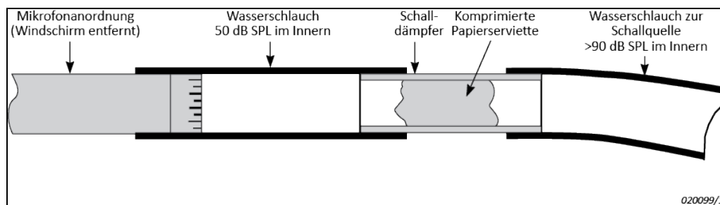
Abb. 3.1 Einrichten der Signalquelle für Prüfung der Störfestigkeit
