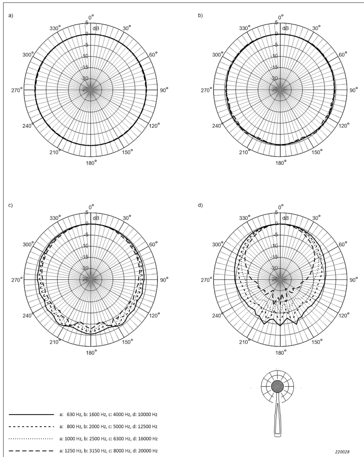
Abb. 4.18 Richtcharakteristik für Windschirm UA-1650, Mikrofon Typ 4966, Mikrofonvorverstärker ZC-0043 und den Schallpegelmesser, wenn der Mikrofonvorverstärker direkt am Schallpegelmesser angebracht ist, in einer zum Display senkrechten Ebene und entlang der Mikrofonachse gemessen. Entspricht Tabelle A.27 bis Tabelle A.29
