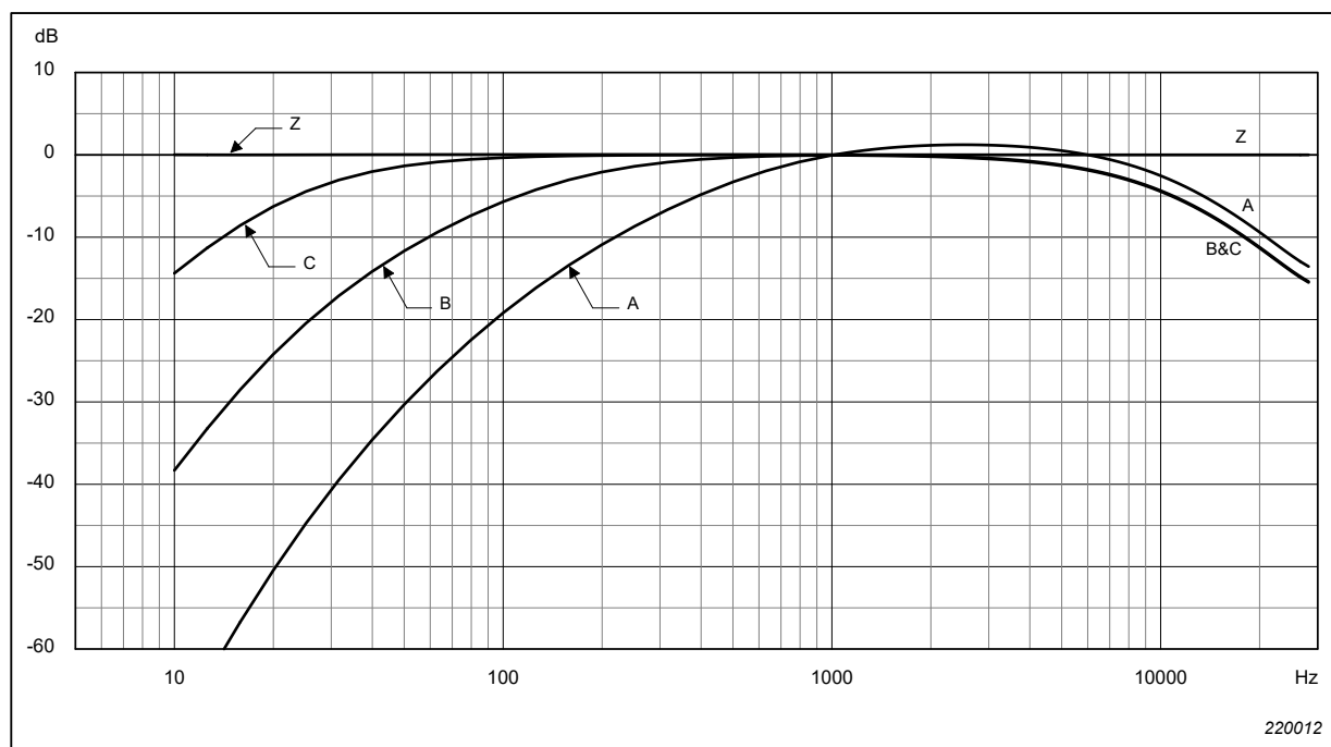
Abb. 4.1 Unkorrigierter elektrischer Frequenzgang, entspricht Tabelle A.1
