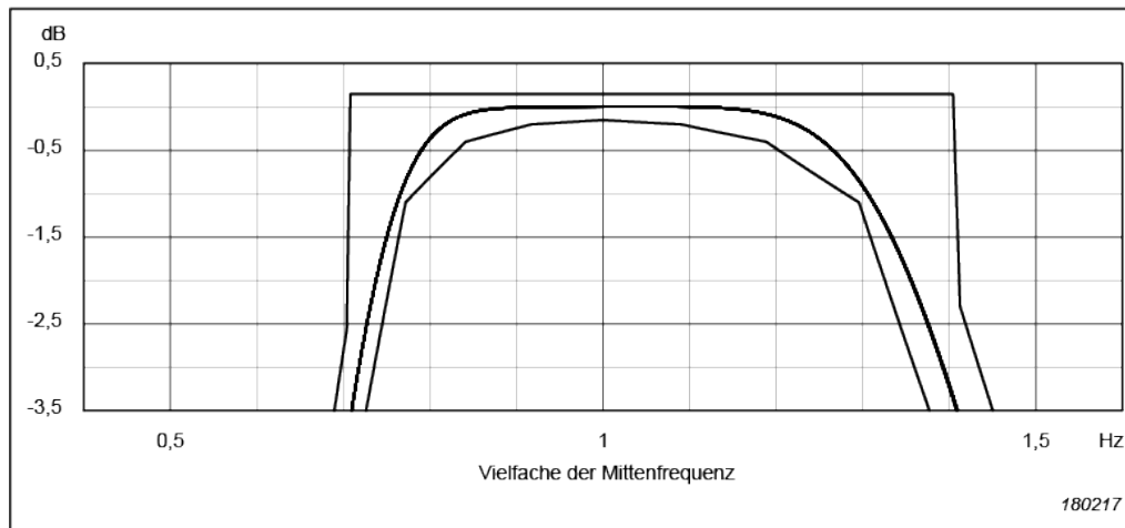
Abb. 4.23 Form der Oktavbandfilter (von 0 bis –3,5 dB). Die innere und äußere Kurve zeigen die Grenzen nach IEC 61260
