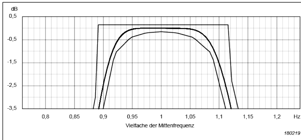
Abb. 4.25 Form der Terzbandfilter (von 0 bis -3,5 dB). Die innere und äußere Kurve zeigen die Grenzen nach IEC 61260
