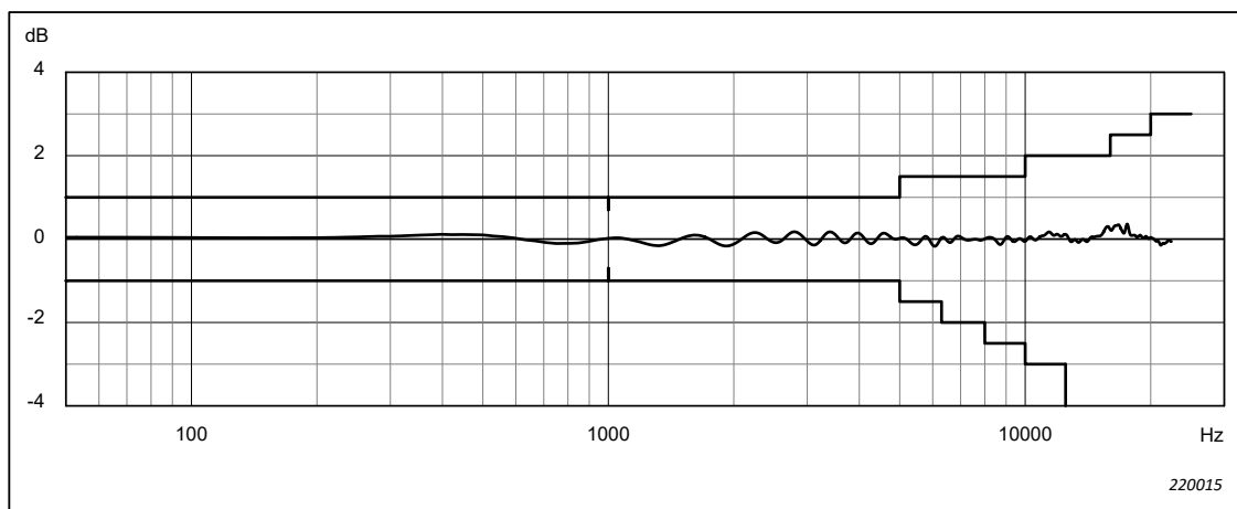
Abb. 4.6 0°-Freifeld-Frequenzgang für Windschirm UA-1650, Mikrofon Typ 4966, Mikrofonvorverstärker ZC-0043 und der elektrische Frequenzgang des Schallpegelmessers, wenn der Mikrofonvorverstärker mit einem Mikrofonverlängerungskabel verbunden ist. Entspricht der Spalte „Akustischer Frequenzgang“ in Tabelle A.4
