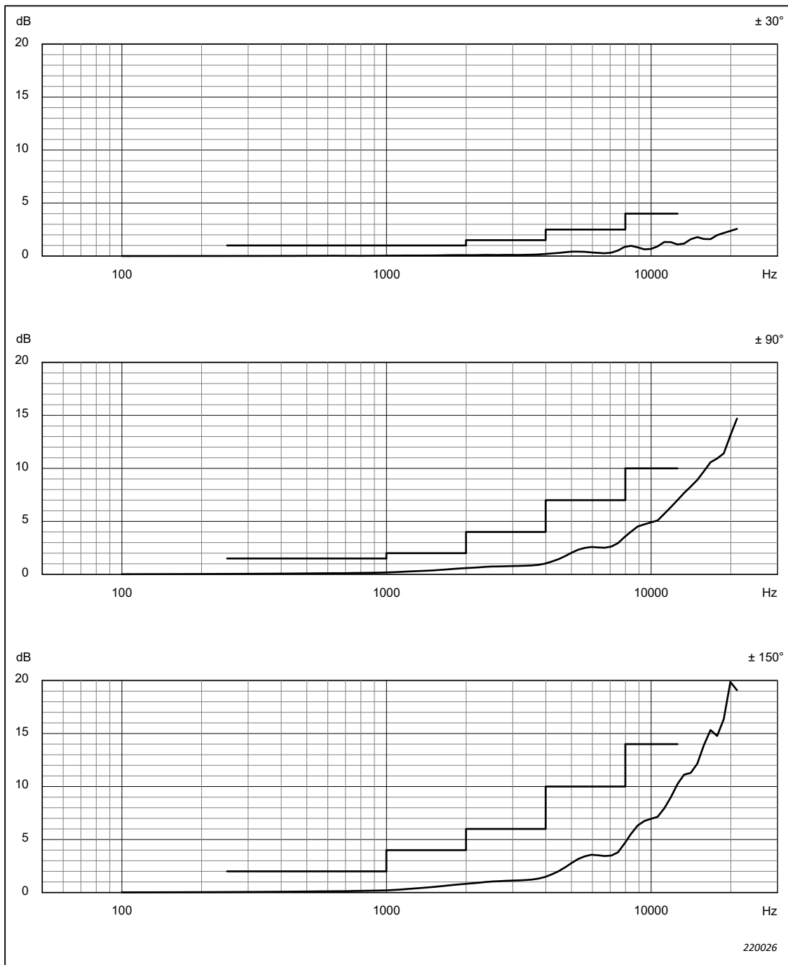
Abb. 4.16 Variationen der Empfindlichkeit für Windschirm UA-1650, Mikrofon Typ 4966 und Mikrofonvorverstärker ZC-0043, wenn der Mikrofonvorverstärker mit einem Mikrofonverlängerungskabel verbunden ist, bei Schalleinfallswinkeln innerhalb von \pm \theta^\circ von der Bezugsrichtung. Entspricht Tabelle A.23
