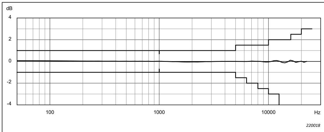
Abb. 4.8 Diffusfeld-Frequenzgang für Mikrofon Typ 4966, Mikrofonvorverstärker ZC-0043 und den Schallpegelmesser mit oder ohne Mikrofonverlängerungskabel am Mikrofonvorverstärker. Entspricht der Spalte „Akustischer Frequenzgang“ in Tabelle A.6
