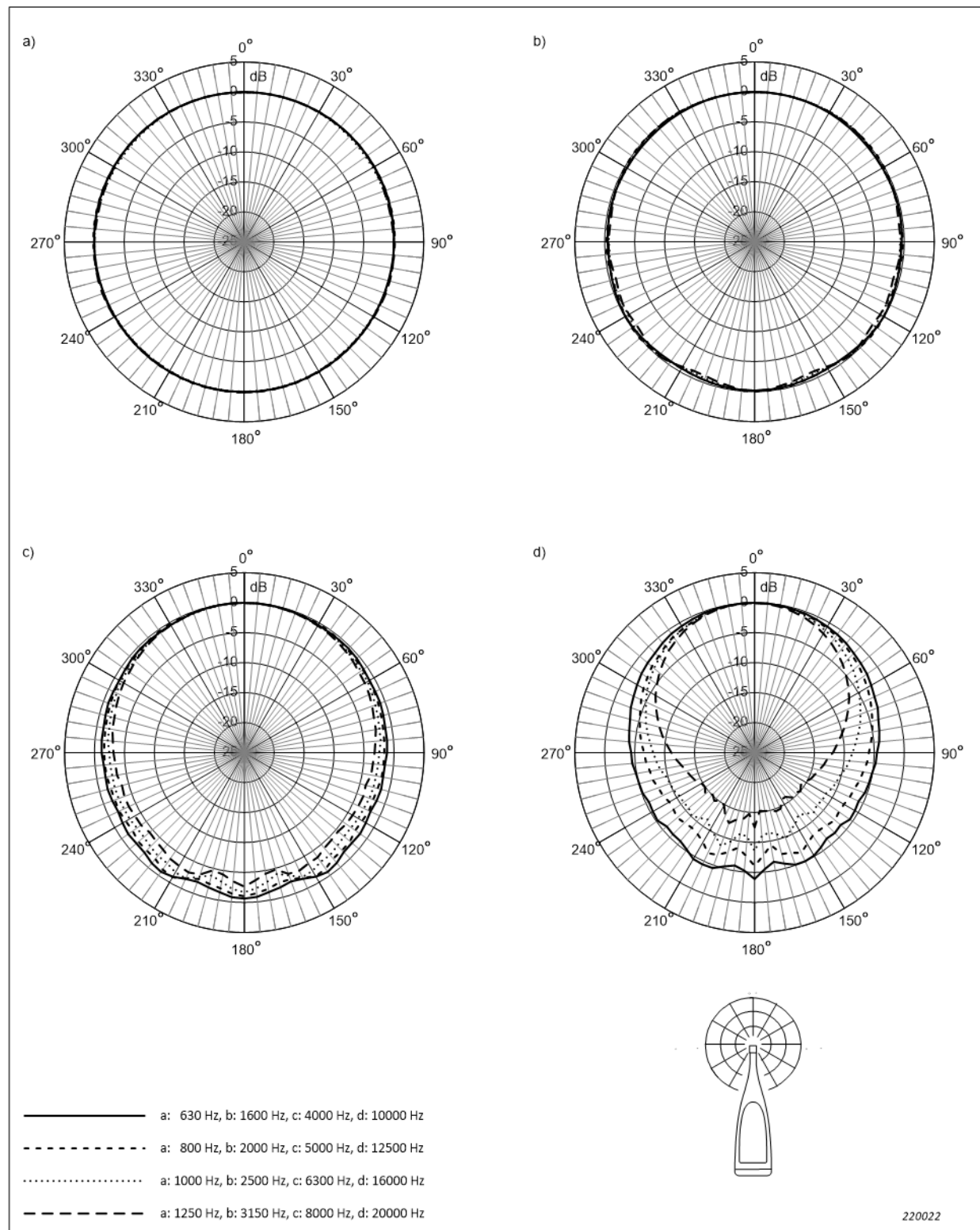
Abb. 4.12 Richtcharakteristik für Mikrofon Typ 4966, Mikrofonvorverstärker ZC-0043 und den Schallpegelmesser, wenn der Mikrofonvorverstärker direkt am Schallpegelmesser angebracht ist, in einer zum Display parallelen Ebene und entlang der Mikrofonachse gemessen. Entspricht Tabelle A.13 bis Tabelle A.15
