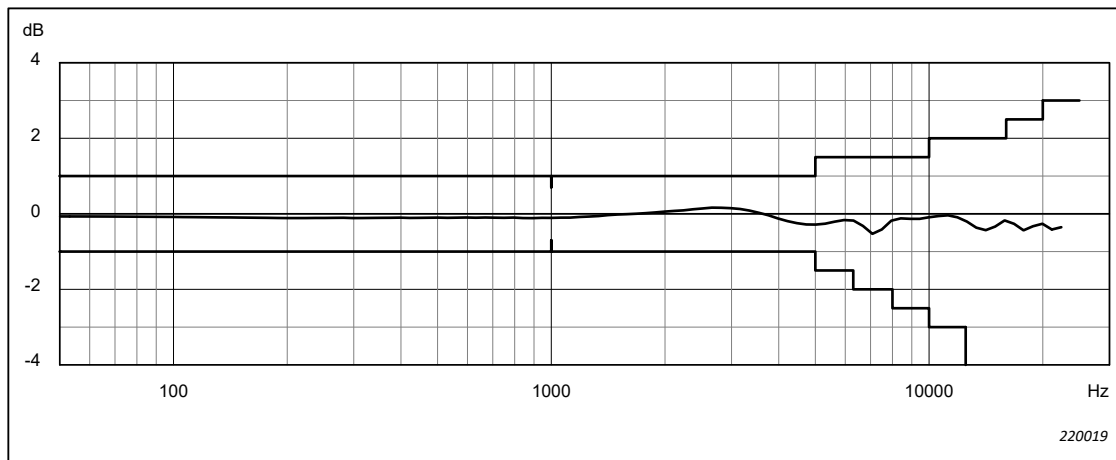
Abb. 4.9 Diffusfeld-Frequenzgang für Windschirm UA-1650, Mikrofon Typ 4966, Mikrofonvorverstärker ZC-0043 und den Schallpegelmesser mit oder ohne Mikrofonverlängerungskabel am Mikrofonvorverstärker. Entspricht der Spalte „Akustischer Frequenzgang“ in Tabelle A.7
