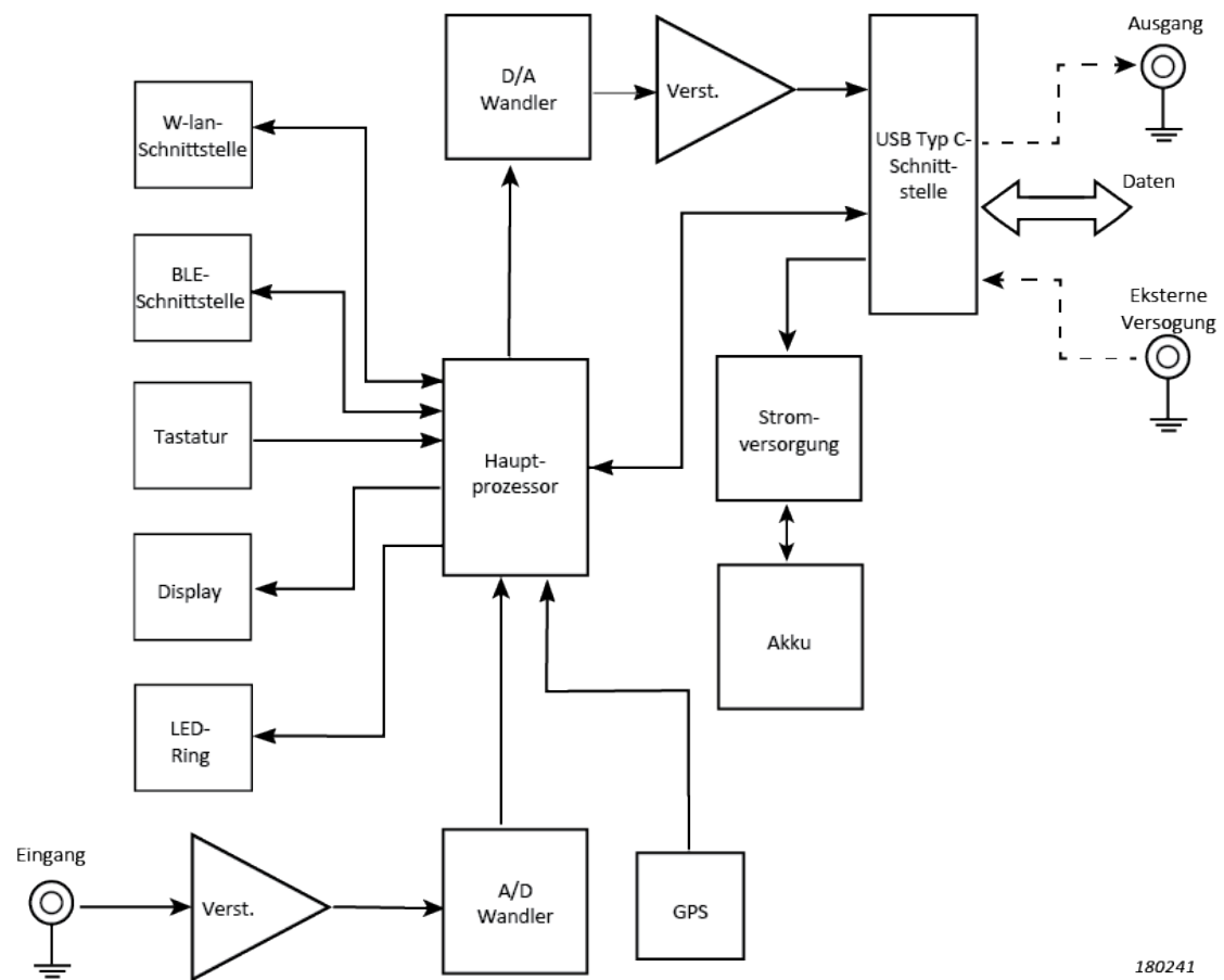
Abb. 1.2 Blockschaltbild für Typ 2255
