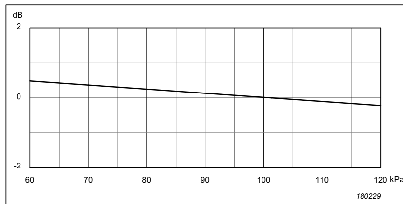
Abb. 2.3 Typische Abweichung der Empfindlichkeit bei 250 Hz vom Wert bei 101,3 kPa als Funktion des Luftdrucks
