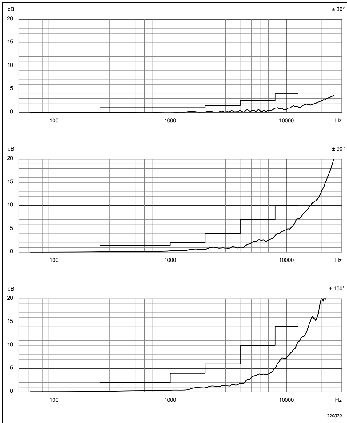
Abb. 4.19 Variationen der Empfindlichkeit von Windschirm UA-1650, Mikrofon Typ 4966, Mikrofonvorverstärker ZC-0043 und dem Schallpegelmesser, wenn der Mikrofonvorverstärker direkt am Schallpegelmesser angebracht ist, bei Schalleinfallswinkeln innerhalb von \pm \theta^\circ von der Bezugsrichtung. Entspricht Tabelle A.30
