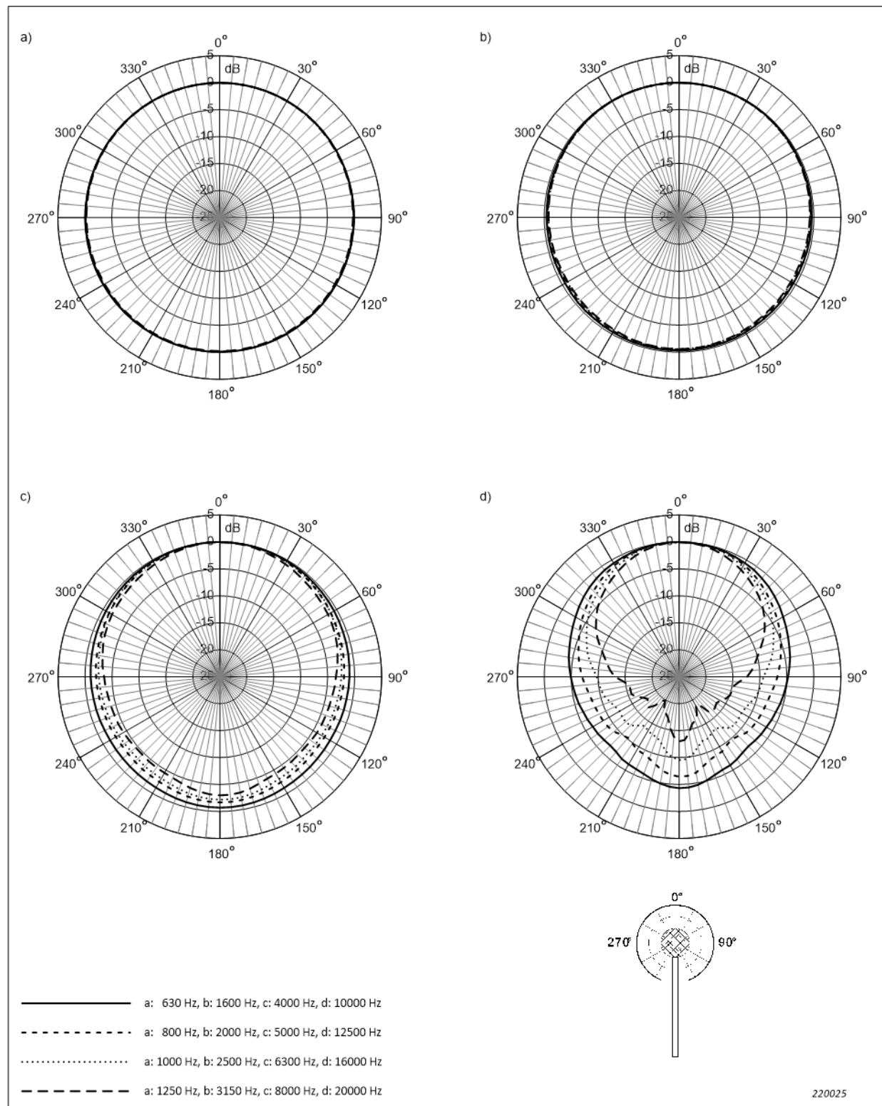
Abb. 4.15 Richtcharakteristik für Windschirm UA-1650, Mikrofon Typ 4966 und Mikrofonvorverstärker ZC-0043, wenn der Mikrofonvorverstärker mit einem Mikrofonverlängerungskabel verbunden ist. Entspricht Tabelle A.20 bis Tabelle A.22
