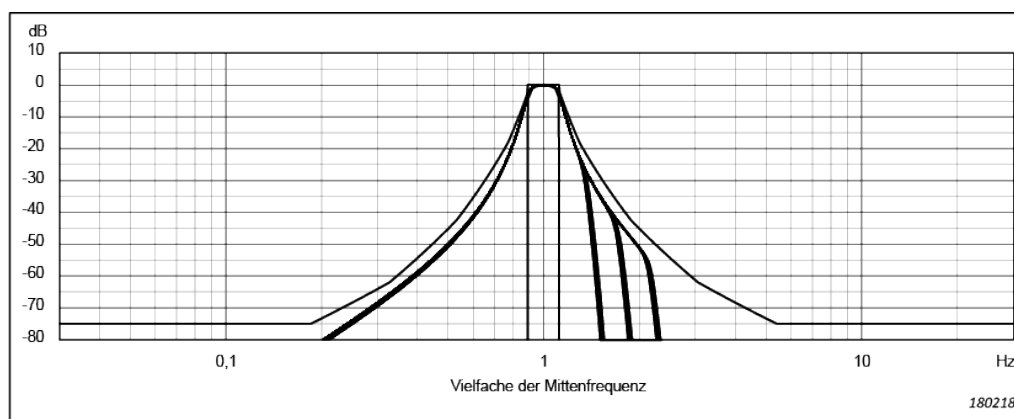
Abb. 4.24 Form der Terzbandfilter (von 0 bis –80 dB). Die innere und äußere Kurve zeigen die Grenzen nach IEC 61260
