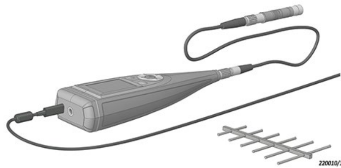
Abb. 3.5 Die Richtung der geringsten Störfestigkeit gegenüber Magnetfeldern mit Netzfrequenz
