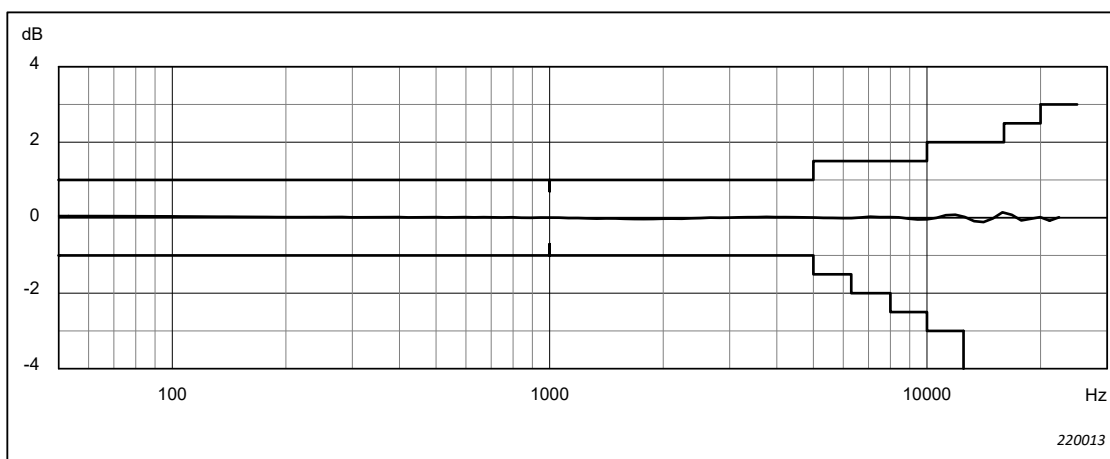
Abb. 4.3 0°-Freifeld-Frequenzgang für Mikrofon Typ 4966, Mikrofonvorverstärker ZC-0043 und der elektrische Frequenzgang des Schallpegelmessers, wenn der Mikrofonvorverstärker mit einem Mikrofonverlängerungskabel verbunden ist. Entspricht der Spalte „Akustischer Frequenzgang“ in Tabelle A.2
