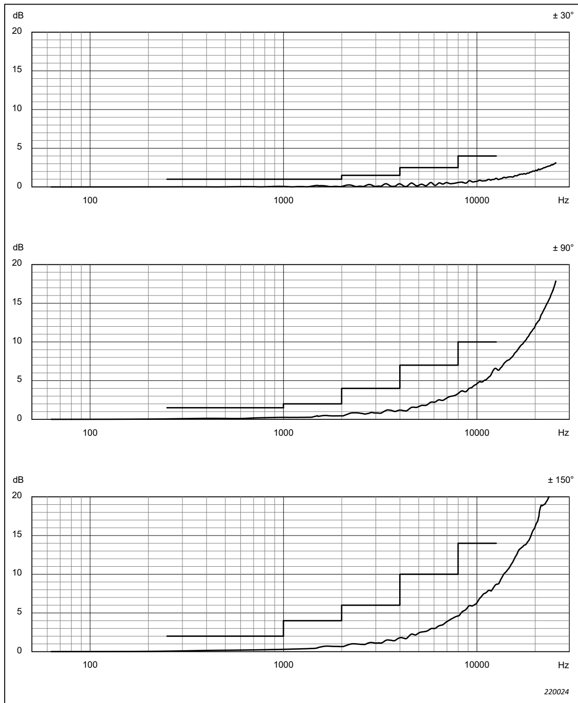
Abb. 4.14 Variationen der Empfindlichkeit für Mikrofon Typ 4966, Mikrofonvorverstärker ZC-0043 und den Schallpegelmesser, wenn der Mikrofonvorverstärker direkt am Schallpegelmesser angebracht ist, bei Schalleinfallswinkeln innerhalb von \pm \theta^\circ von der Bezugsrichtung. Entspricht Tabelle A.19
