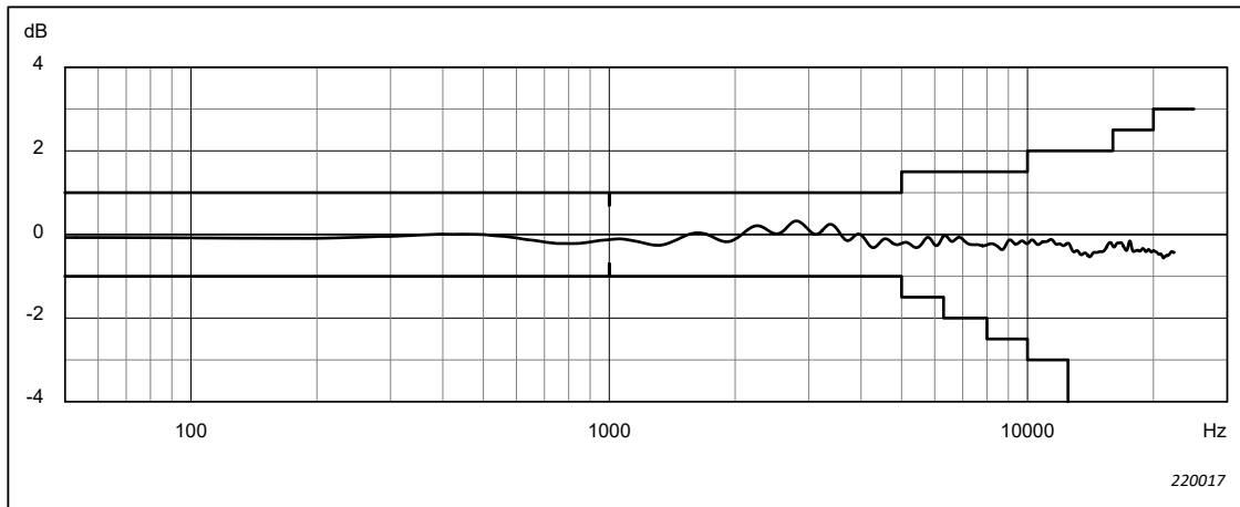
Abb. 4.7 0°-Freifeld-Frequenzgang für Windschirm UA-1650, Mikrofon Typ 4966, Mikrofonvorverstärker ZC-0043 und den Schallpegelmesser, wenn der Mikrofonvorverstärker direkt am Schallpegelmesser angebracht ist. Entspricht der Spalte „Akustischer Frequenzgang“ in Tabelle A.5
