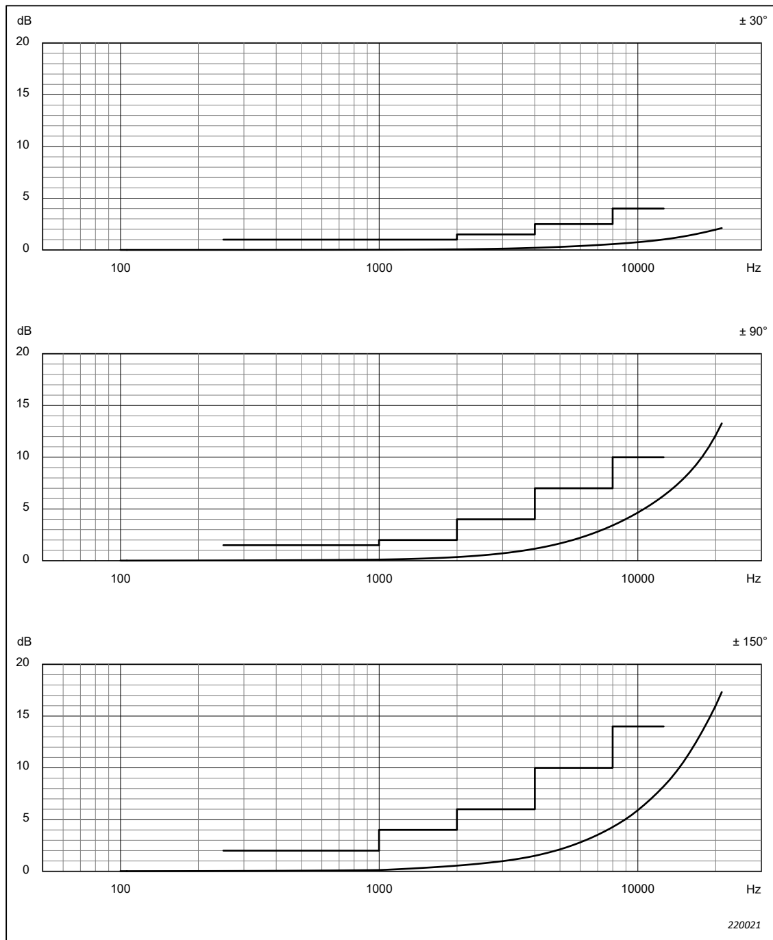
Abb. 4.11 Variationen der Empfindlichkeit für Mikrofon Typ 4966 und Mikrofonvorverstärker ZC-0043, wenn der Mikrofonvorverstärker mit einem Mikrofonverlängerungskabel verbunden ist, bei Schalleinfallswinkeln innerhalb von \pm \theta^\circ von der Bezugsrichtung. Entspricht Tabelle A.12
