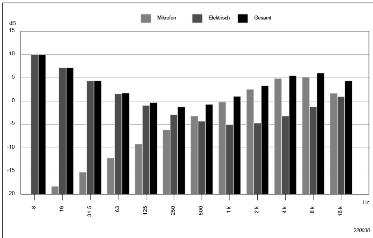
Abb. 4.20 Typisches Eigenrauschen, Oktavband
