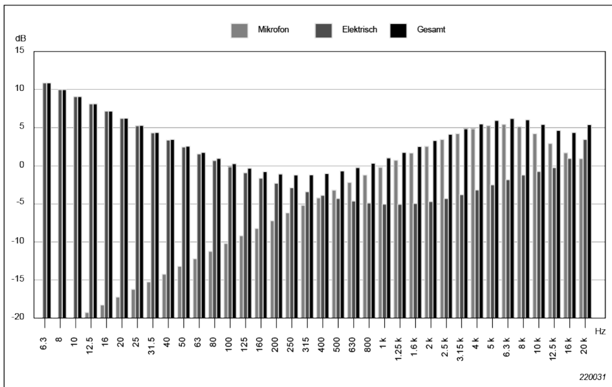
Abb. 4.21 Typisches Eigenrauschen, Terzband
