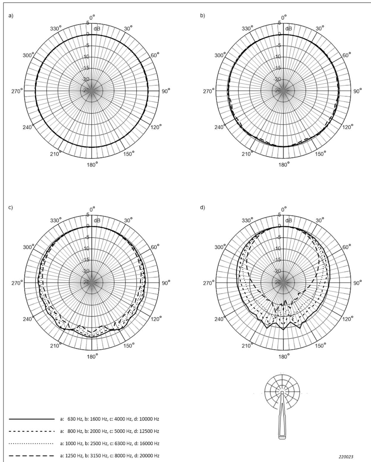
Abb. 4.13 Richtcharakteristik für Mikrofon Typ 4966, Mikrofonvorverstärker ZC-0043 und den Schallpegelmesser, wenn der Mikrofonvorverstärker direkt am Schallpegelmesser angebracht ist, in einer zum Display senkrechten Ebene und entlang der Mikrofonachse gemessen. Entspricht Tabelle A.16 bis Tabelle A.18
