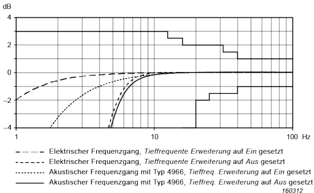
Abb. 4.2 Typische Frequenzgänge bei niedrigen Frequenzen
