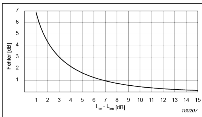
Abb. 2.1 Fehler durch Eigenrauschen
