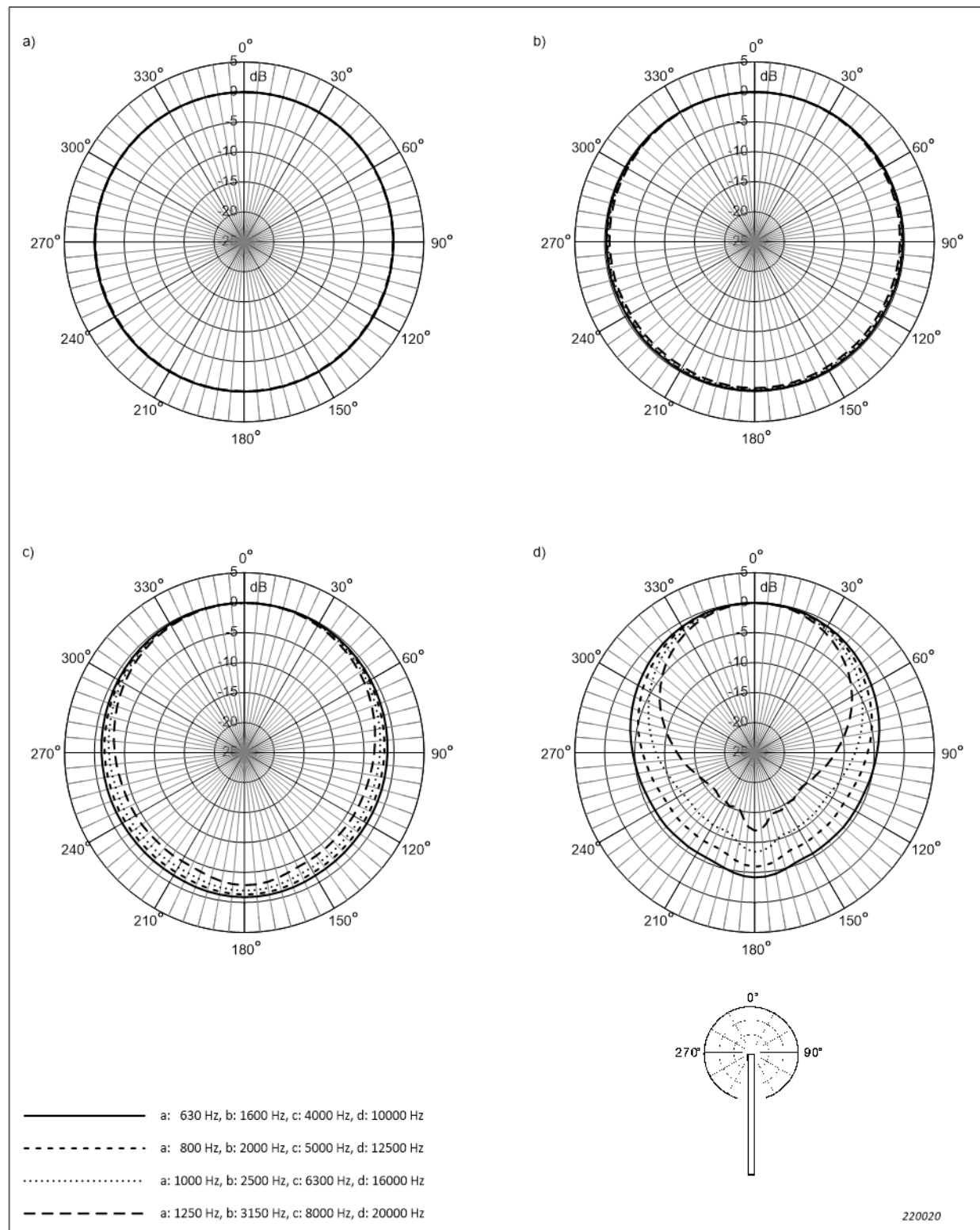
Abb. 4.10 Richtcharakteristik für Mikrofon Typ 4966 und Mikrofonvorverstärker ZC-0043, wenn der Mikrofonvorverstärker mit einem Mikrofonverlängerungskabel verbunden ist. Entspricht Tabelle A.9 bis Tabelle A.11
