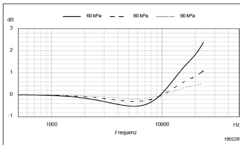
Abb. 2.2 Typische Abweichung des Frequenzgangs (normalisiert bei 250 Hz) vom Wert bei 101,3 kPa als Funktion von Luftdruckänderungen
