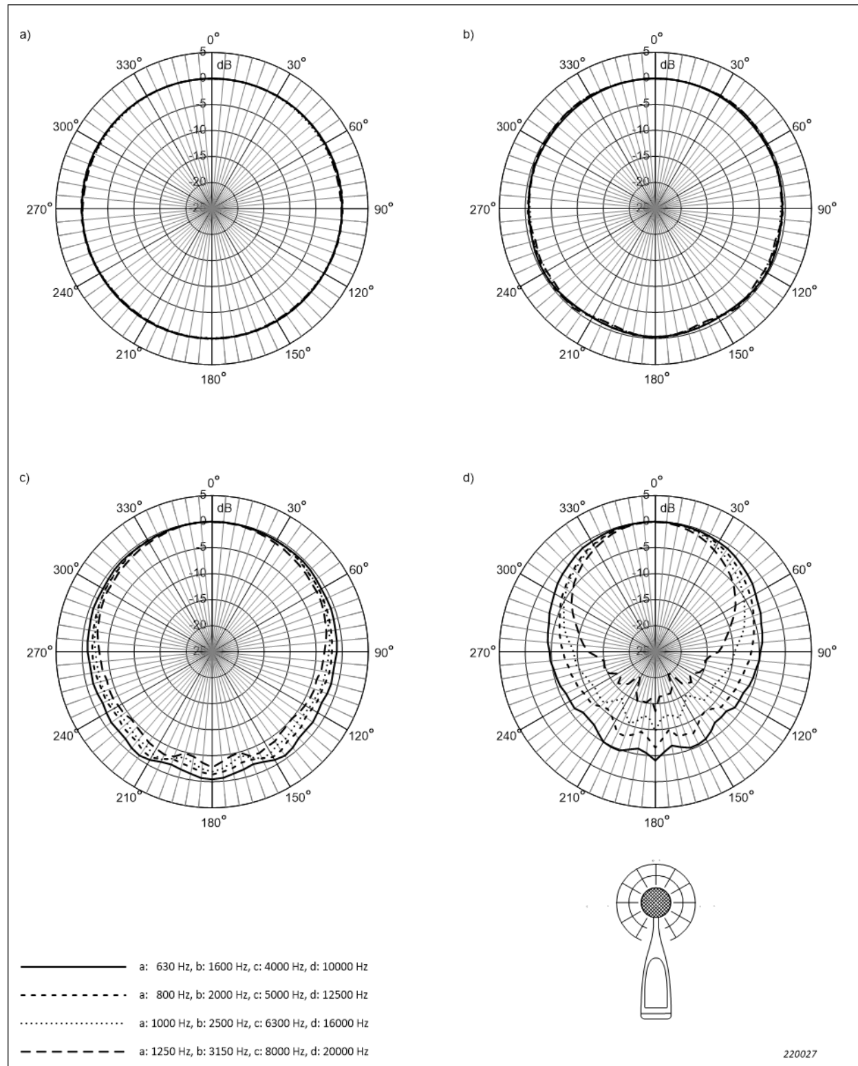
Abb. 4.17 Richtcharakteristik für Windschirm UA-1650, Mikrofon Typ 4966, Mikrofonvorverstärker ZC-0043 und den Schallpegelmesser, wenn der Mikrofonvorverstärker direkt am Schallpegelmesser angebracht ist, in einer zum Display parallelen Ebene und entlang der Mikrofonachse gemessen. Entspricht Tabelle A.24 bis Tabelle A.26
